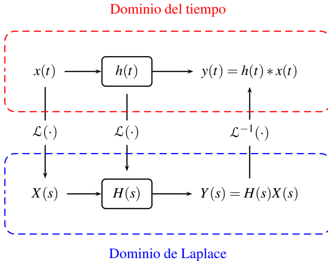
Figura 1.5: Función de transferencia y su relación con la entrada y la salida en el dominio del tiempo y en el dominio de Laplace.
