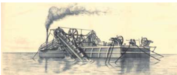
Vista de una de las dragas destinadas a la limpia del Puerto del Grao de Valencia en Revista de Obras Públicas , 1854. Xilografía a la contrafibra. ©Autoridad Portuaria de València.
